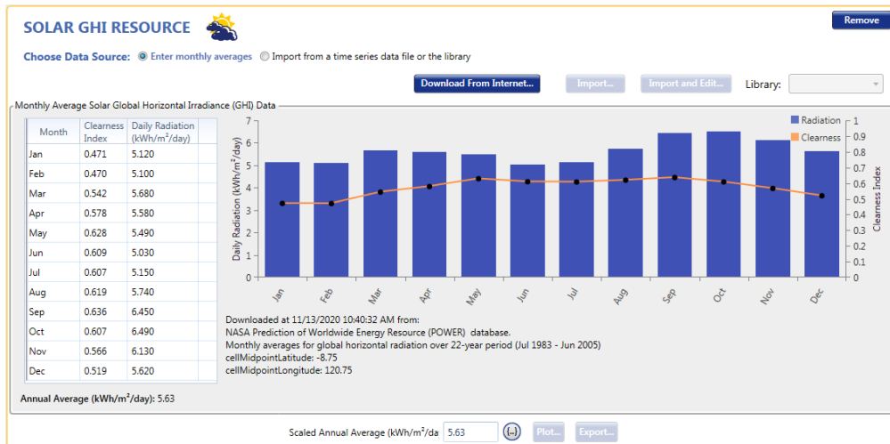
Gambar 3. Potensi energi surya di Desa Koak
