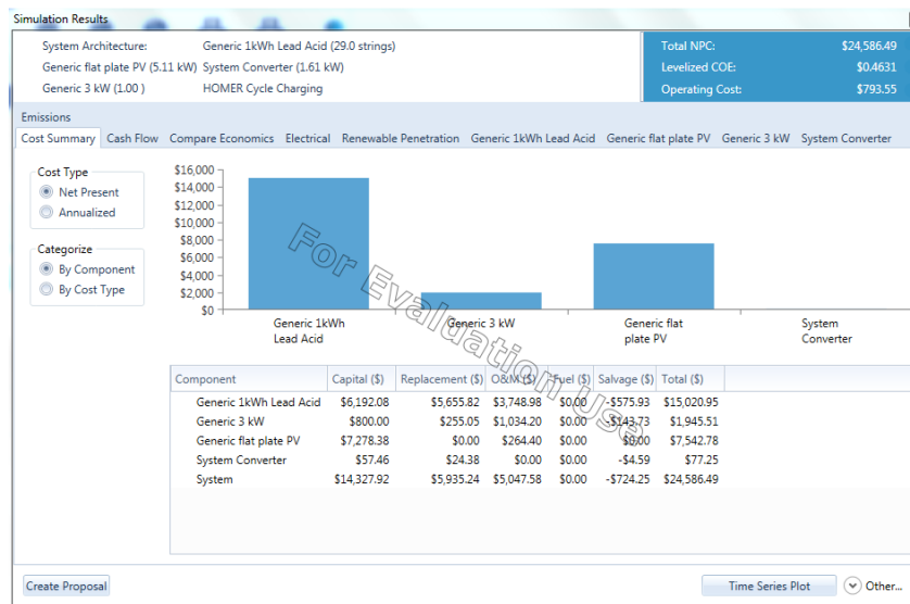
Gambar 11. Biaya yang dibutuhkan oleh sistem
