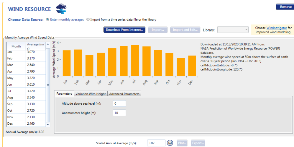
Gambar 4. Potensi energi angin di Desa Koak
