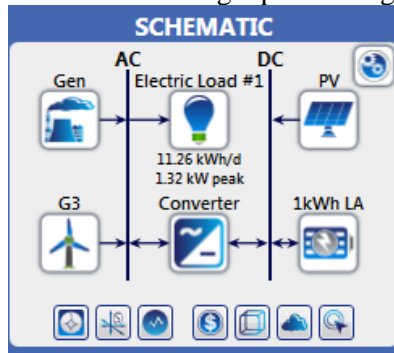
Gambar 8. Konfigurasi komponen dalam simulasi
